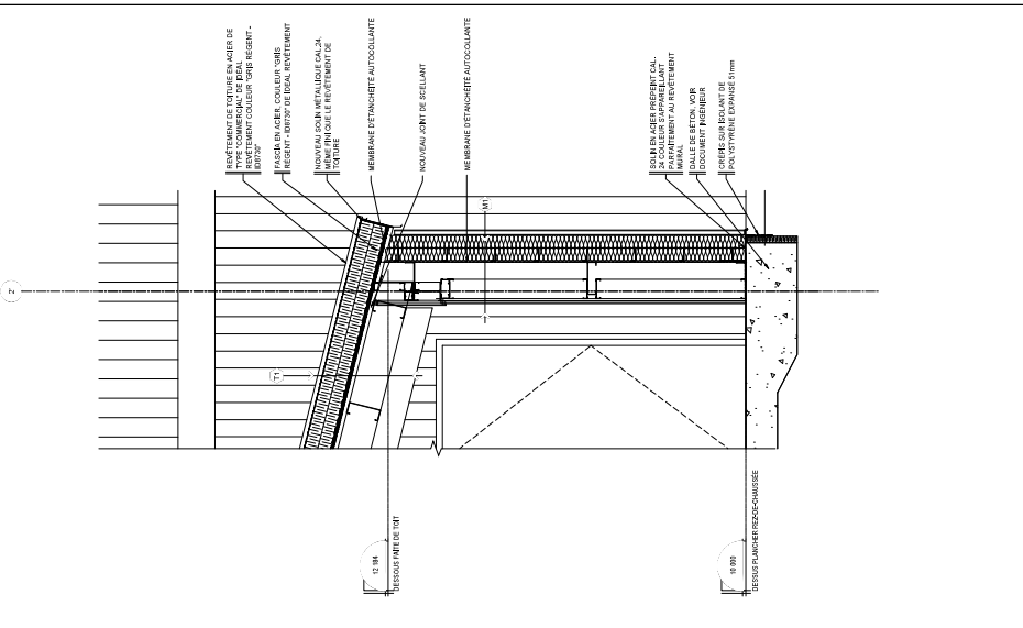
COUPE DE MUR TYPE 1
