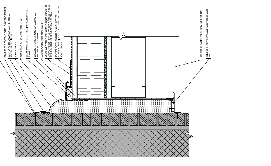
COUPE DE MUR TYPE 3
