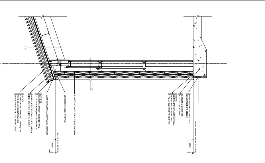
COUPE DE MUR TYPE 2
